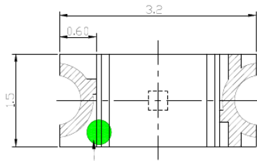
负极标志 Cathode Mark
