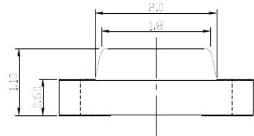
负极标志 Cathode Mark
