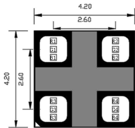
主视图 Main view
