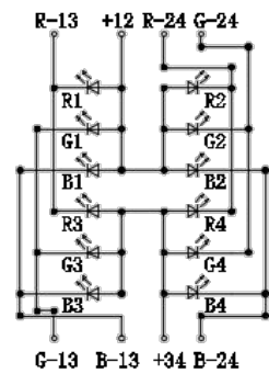
极性 Polarity
