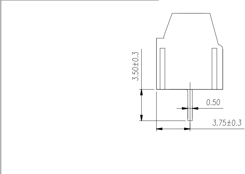
P.C.B. LAYOUT
