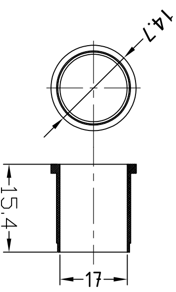
C, 密封圈
