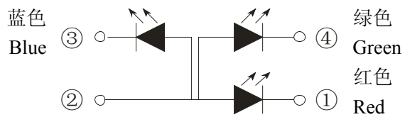
极性 Polarity
