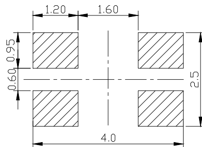
推荐焊盘
