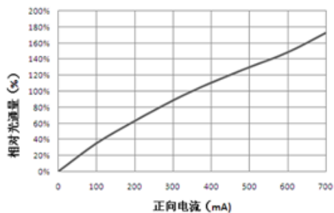
■ 正向电流—相对光通量曲线图
