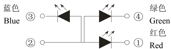
极性 Polarity
