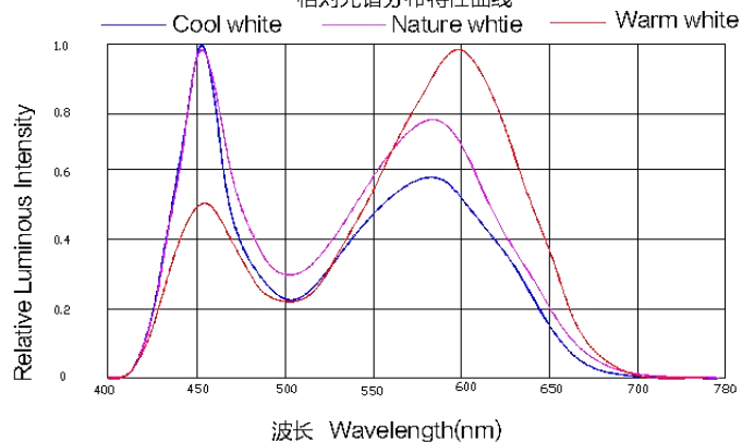
相对光谱分布特性曲线
