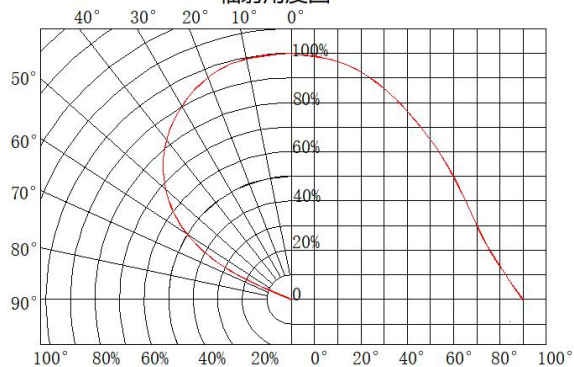
辐射角度图
