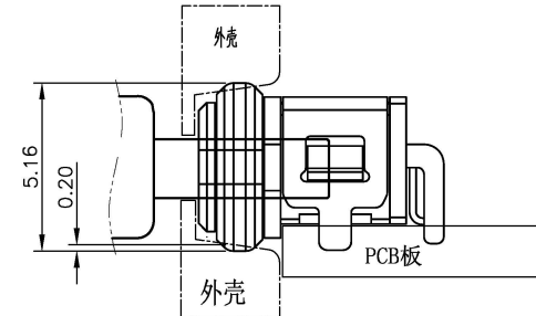
组装示意图
